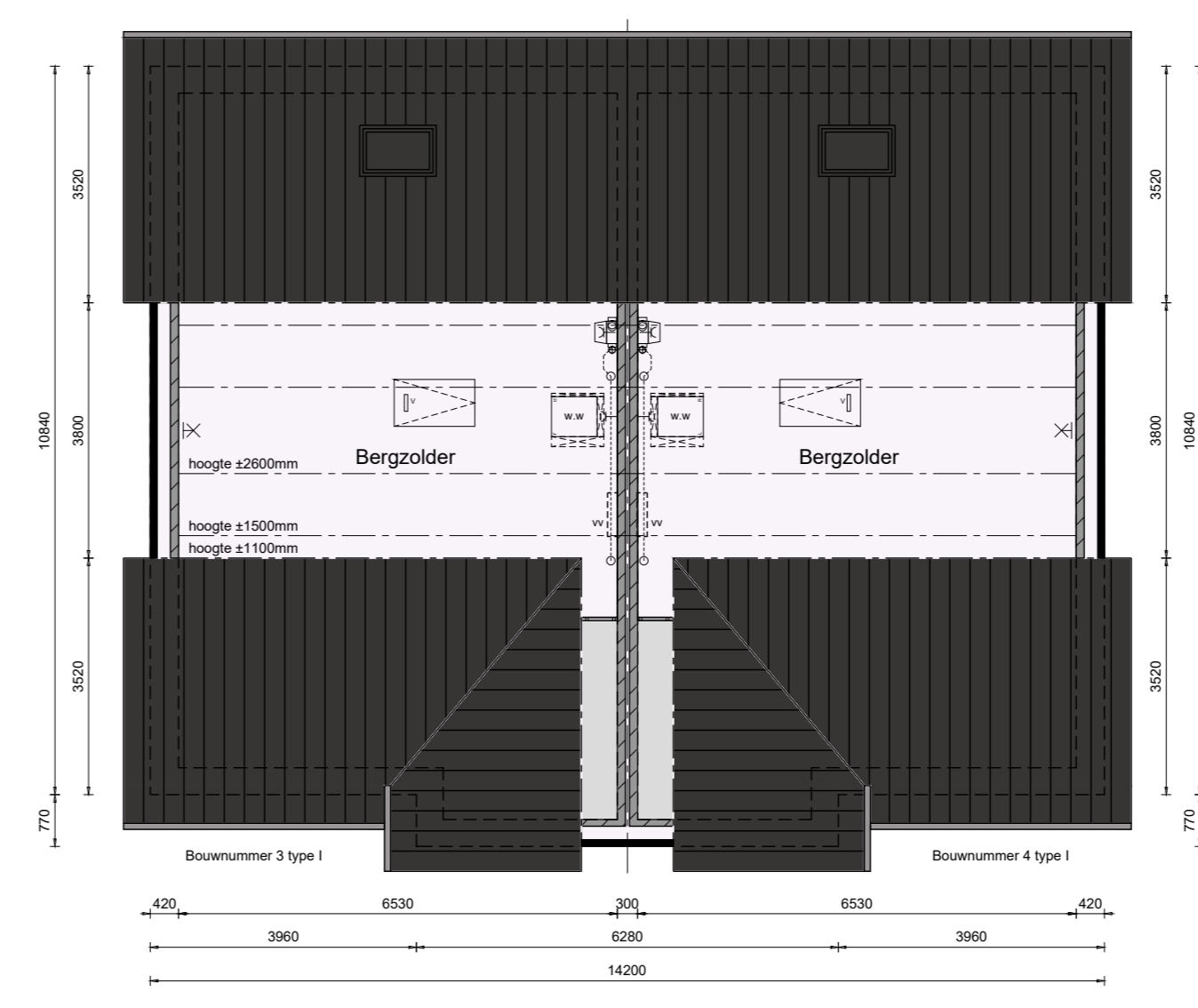
v.z.v. vloerverwarming
