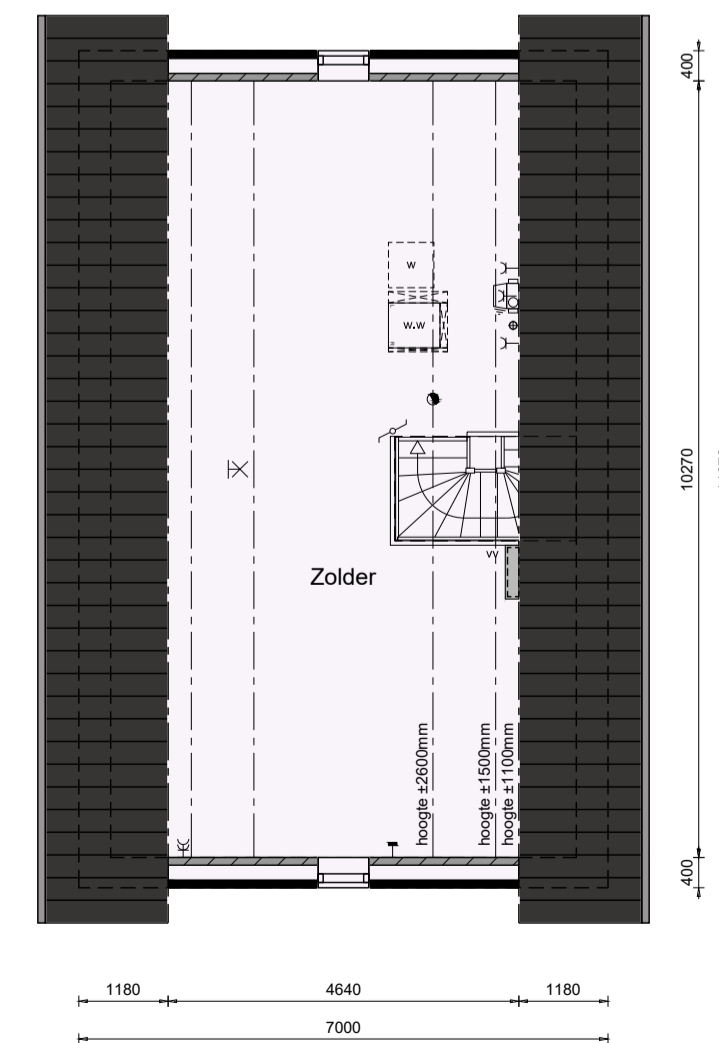
v.z.v. vloerverwarming
